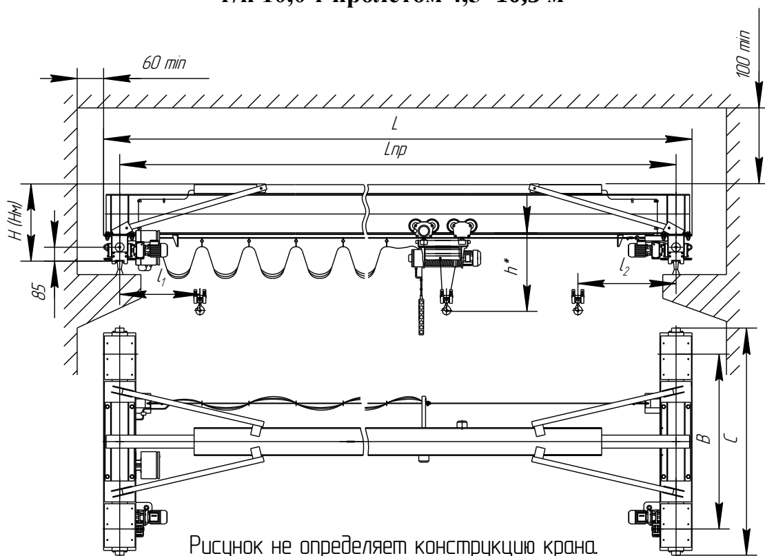
Рис. 1 Общий вид крана
