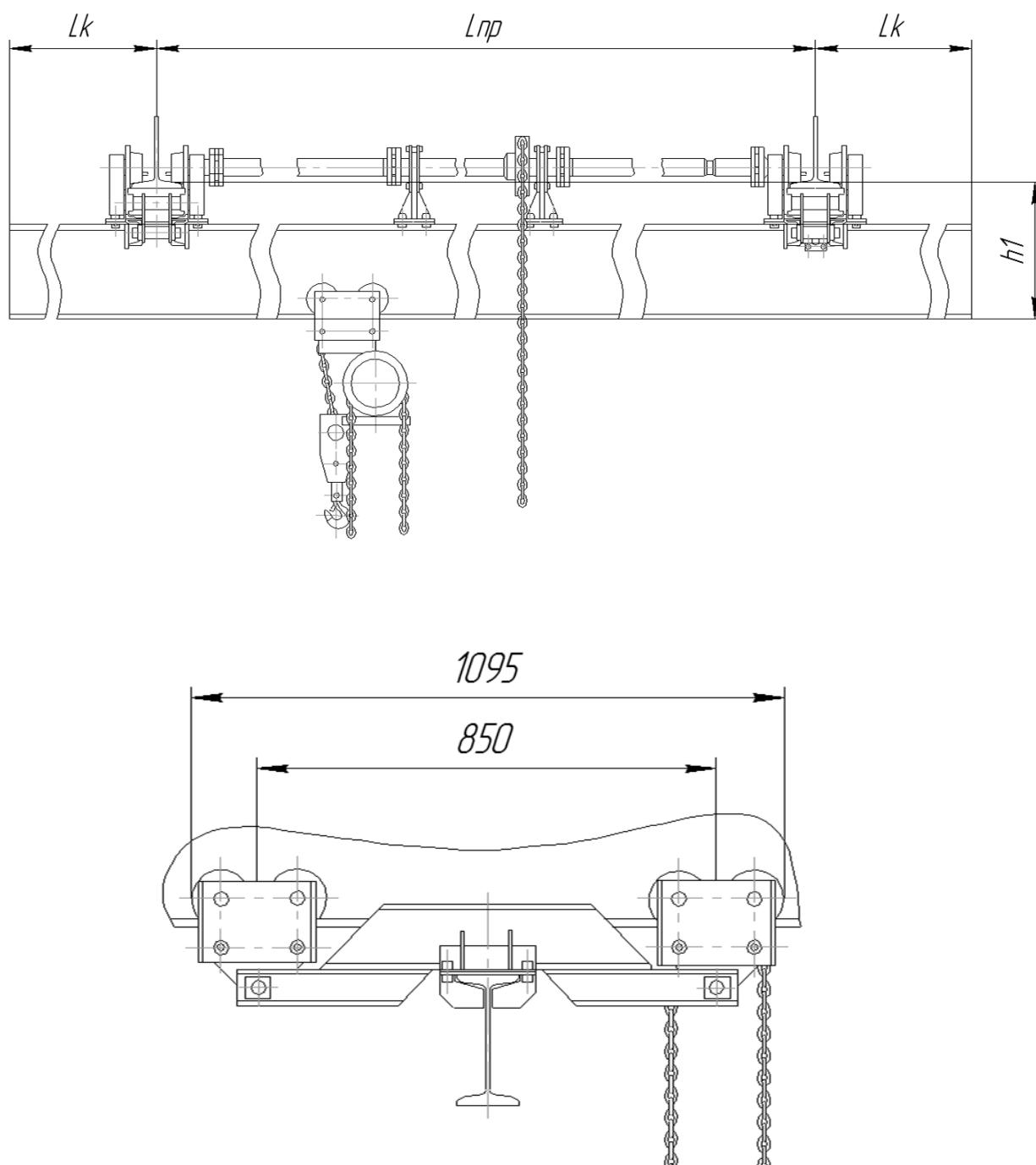
Рис. 1 Общий вид крана
