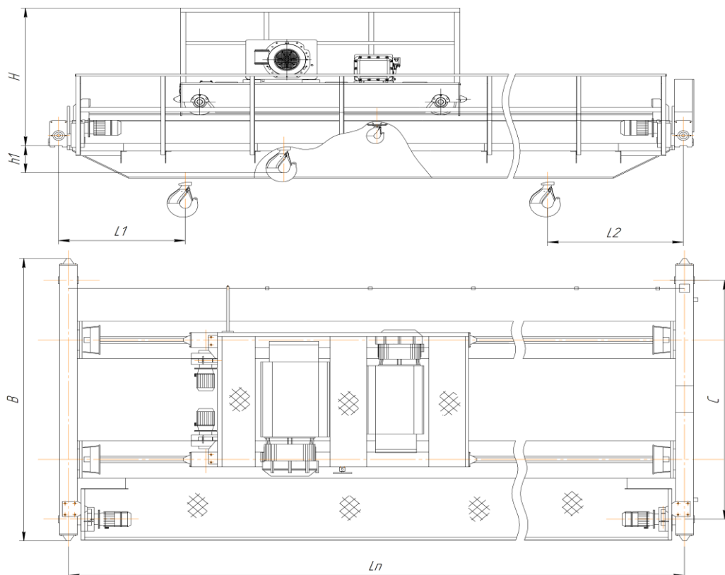
Технические характеристики и размеры крана
